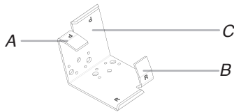
A. Gancho P B. Gancho R C. Soporte P y R
