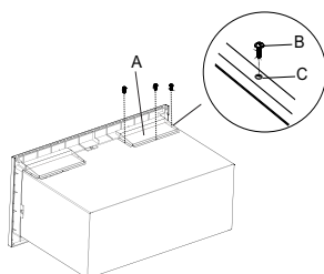
A. Conducto de enfriamiento del lado izquierdo B. Tornillos cortos (3) C. Orificio para tornillo (3)
